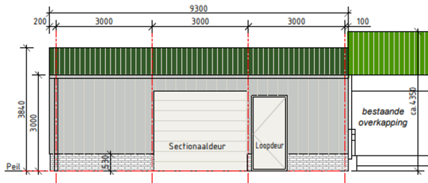
Vooraanzicht materiaalloods
