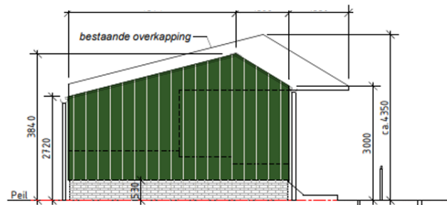
Zijaanzicht materiaalloods
